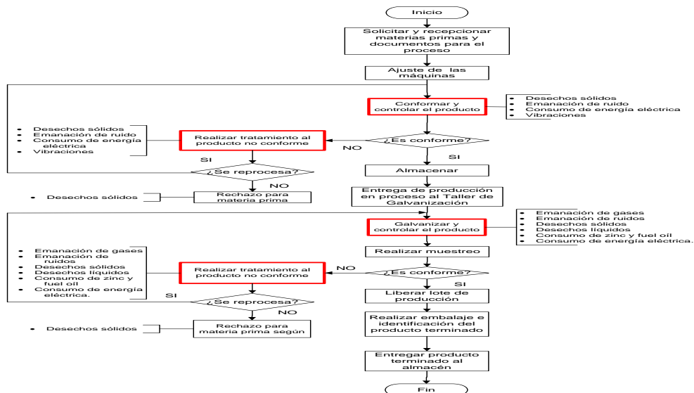
Figura 3: Diagrama de Flujo del proceso de producción Fuente: Elaboración Propia
